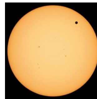
Venus Transit
