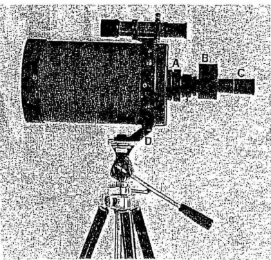
The Porro Prism (A) Visual back (B) Porro Prism (C) Ocular (D) C5 photo tripod adapter
